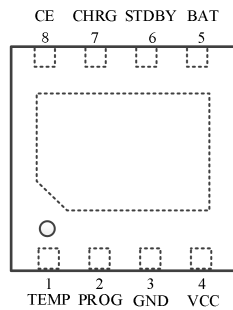
DFN2*2-8封装，散热片接地
