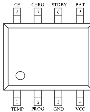
ESOP-8封装，散热片接地
